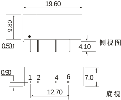
引脚方式
